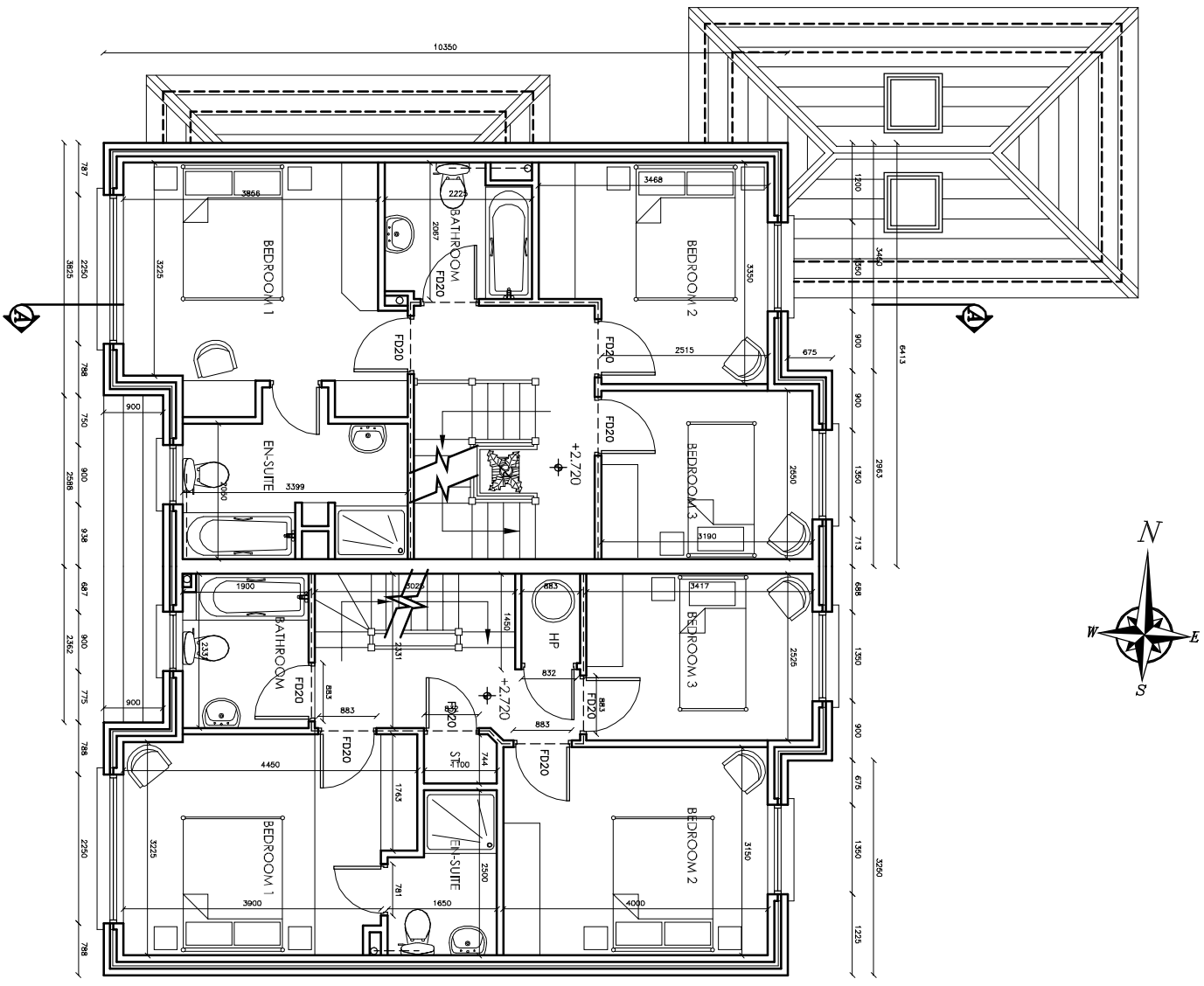
HOUSE TYPE F1 FIRST FLOOR PLAN
